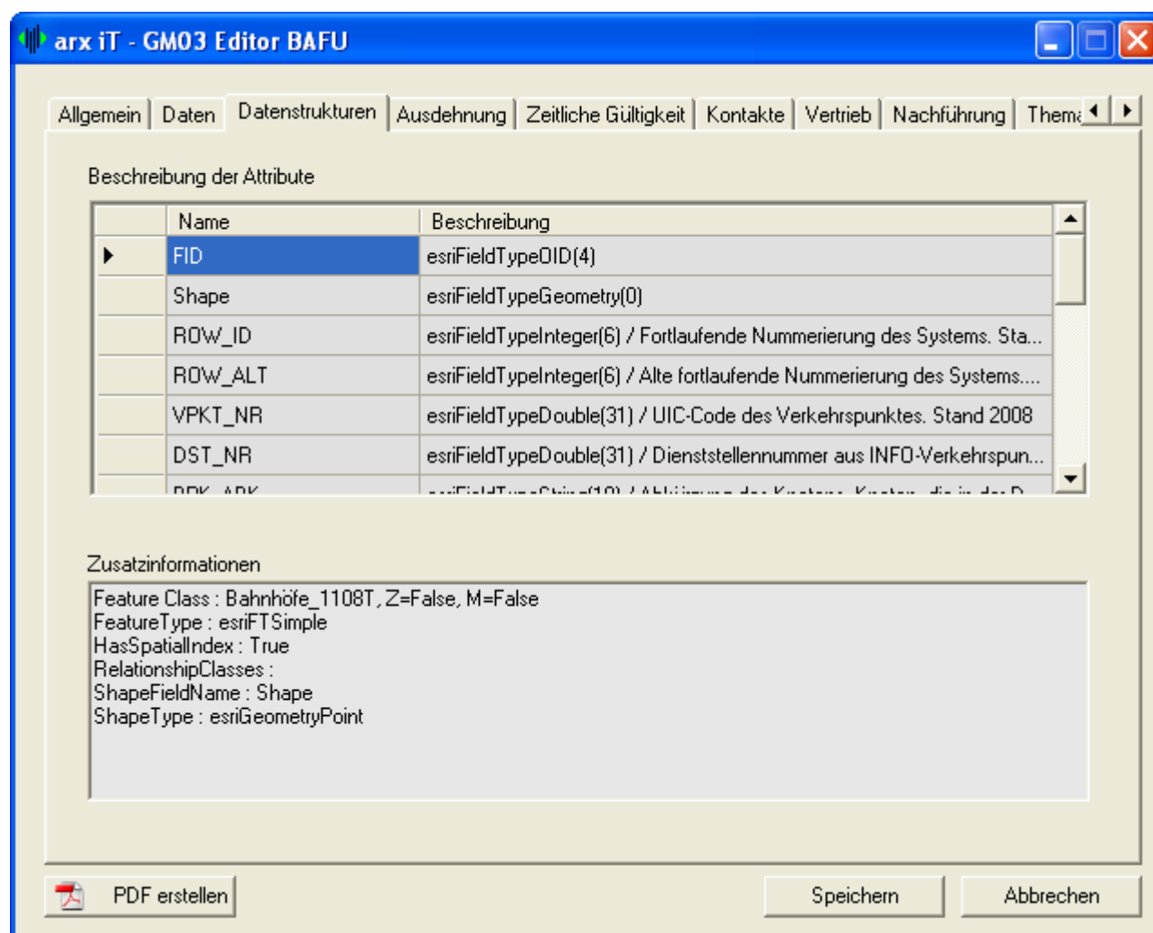
Abbildung 15: TAB Datenstrukturen
