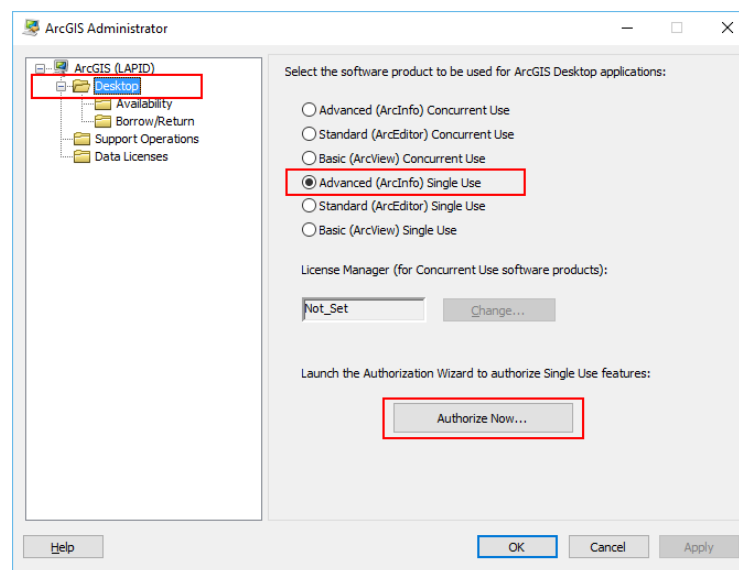
Abb. 1: Autorisierungsoptionen
