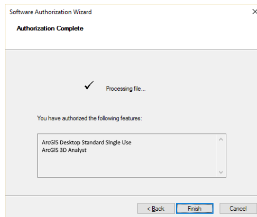
Abb. 9: Autorisierung abgeschlossen
