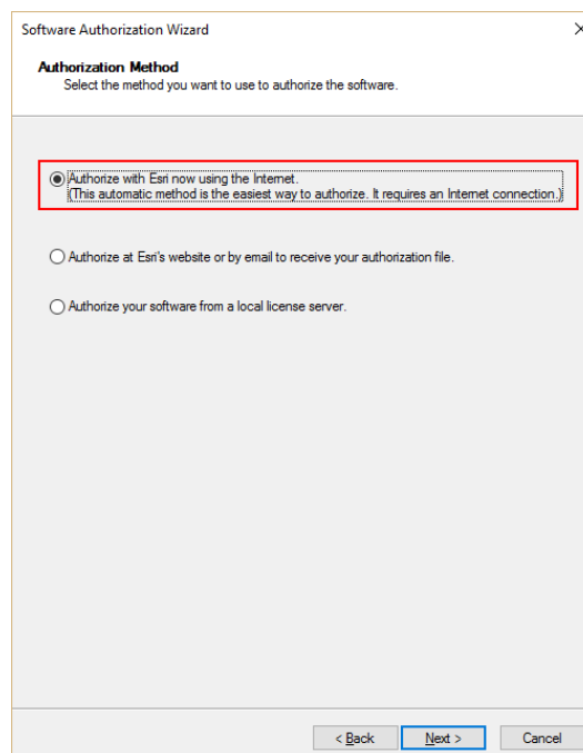
Abb. 3: Autorisierungsmethoden
